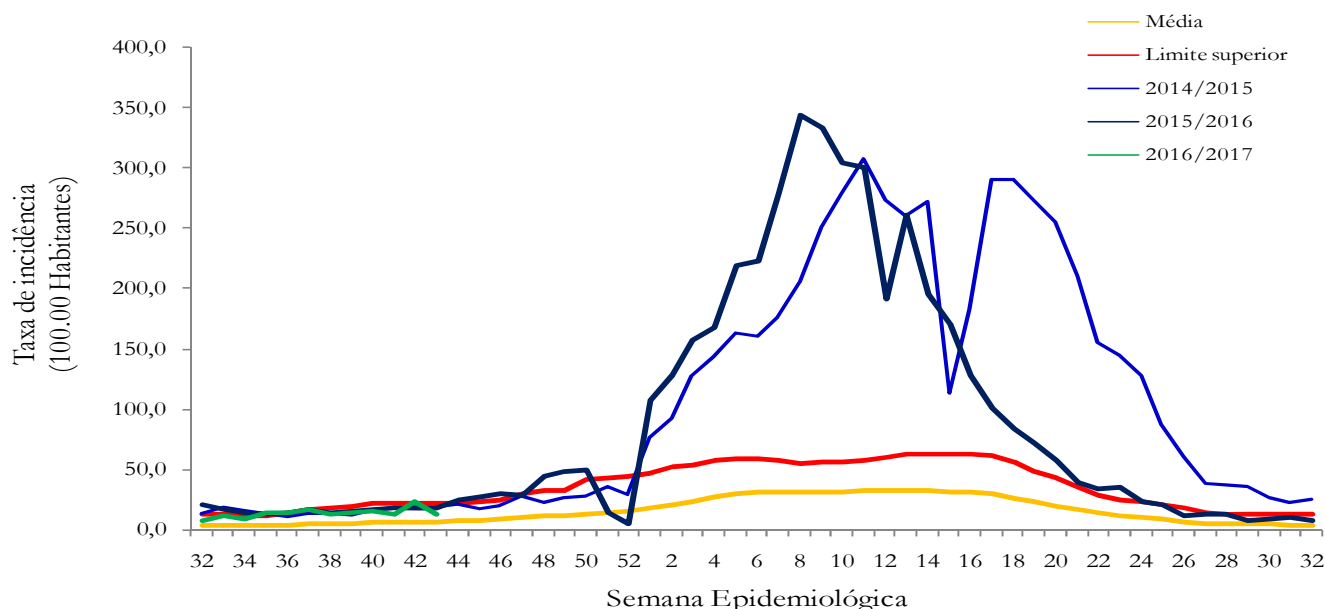
Gráfico 1 – Diagrama de Controle da dengue em Goiânia 2014-2016*
